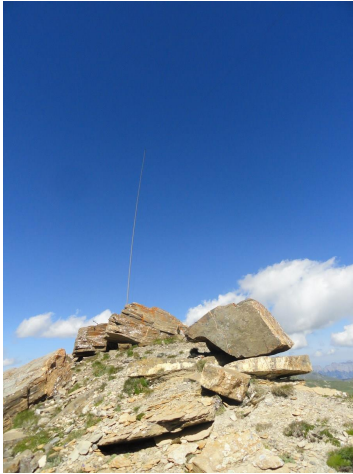
Wissgandstöckli: Mast in den Felsblöcken einklemmen. EndfeedZ gut zum Steinmannli hin verspannbar. Kein Kreuz!.
